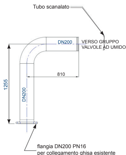
TUBO DI COLLEGAMENTO DELL'ALIMENTAZIONE IDRICA PER VALVOLE AD UMIDO (4x) non valida per l'esecuzione
